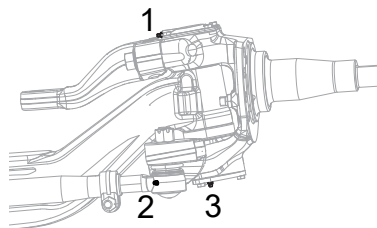
Illustration 67 : Points de graissage pour essieu avant FX-20 PACCAR
