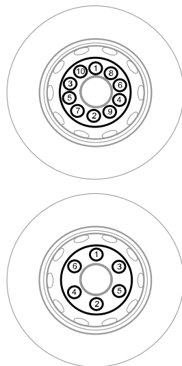
Illustration 70 : Roues à disque centrées par goujons
