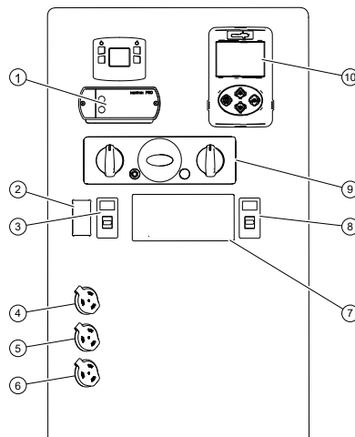
Illustration 33 : Panneau de commande du compartiment couchette
