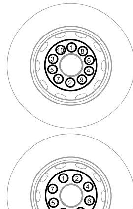
Illustration 69 : Roues à disque centrées par moyeu
