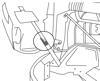
Illustration 11 : Dispositif de fixation du capot
