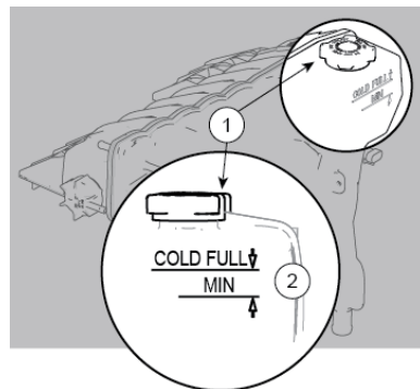
Illustration 62 : Réservoir d'équilibre de liquide de refroidissement monté sur cloison
